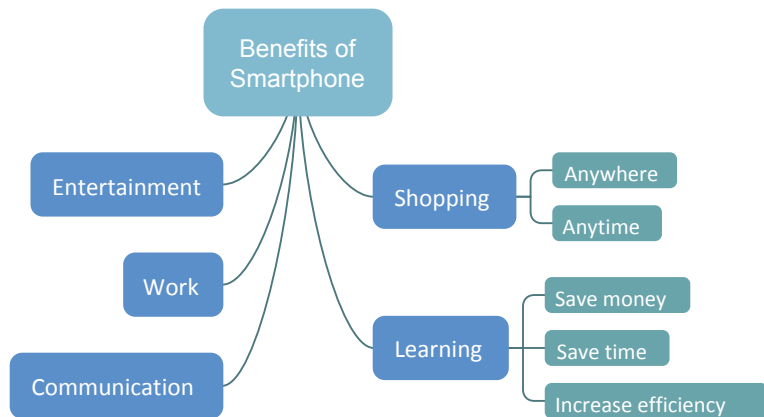
Mind Map
