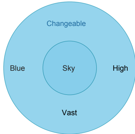
Circle Diagram
